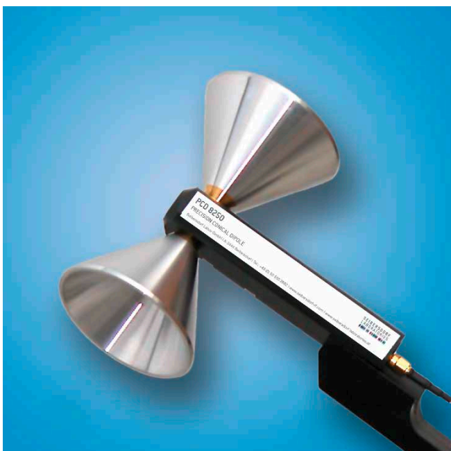
PCD 8250 antenna
